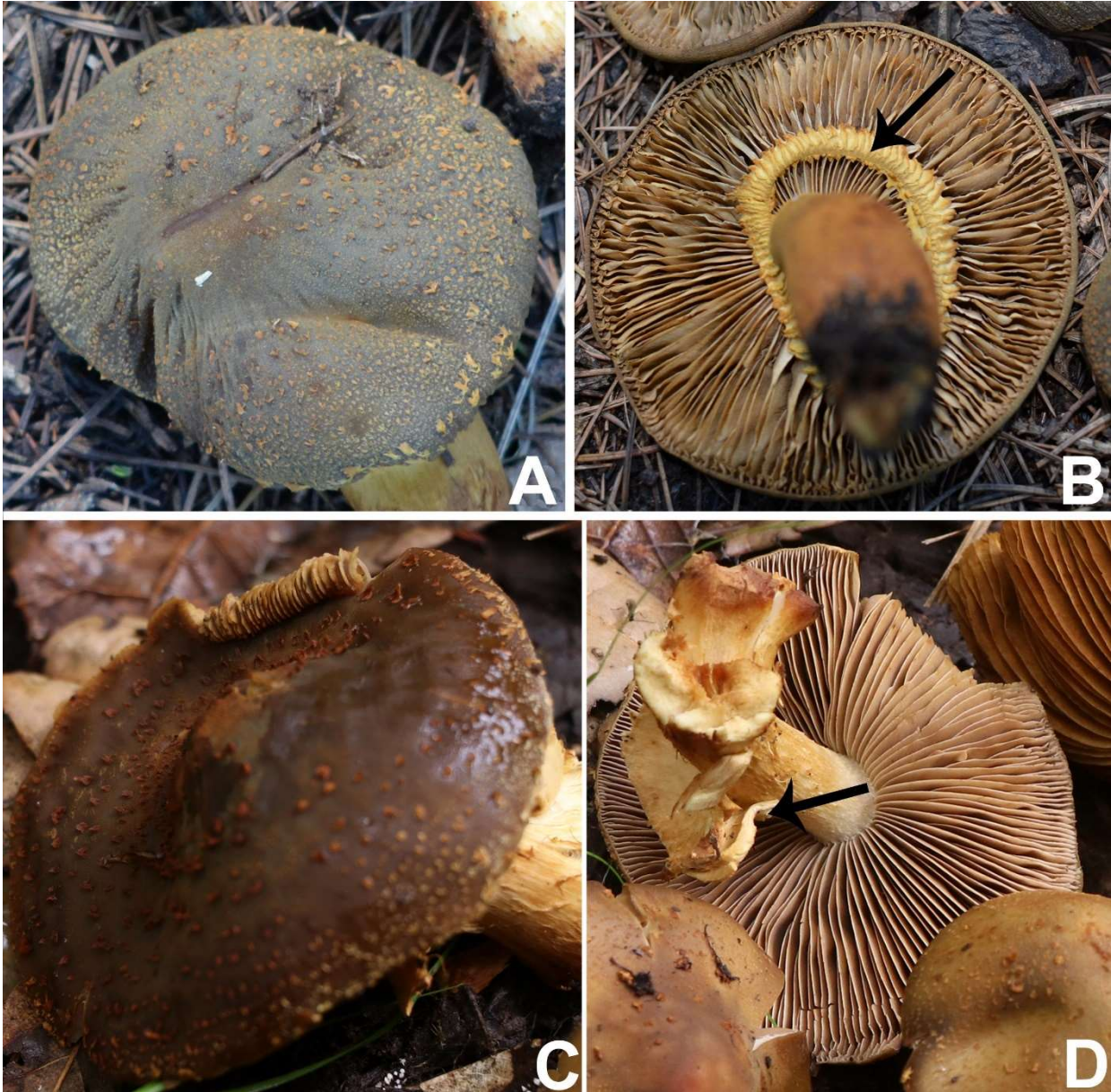
Fig S1. Comparison of Descolea flavoannulata (A & B) and D. indoquercina (C & D). A. & C. Pileal and B. & D. Lamellar.
